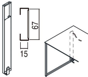
ソリスト 配線立上げダクト フレーム脚用 720H
