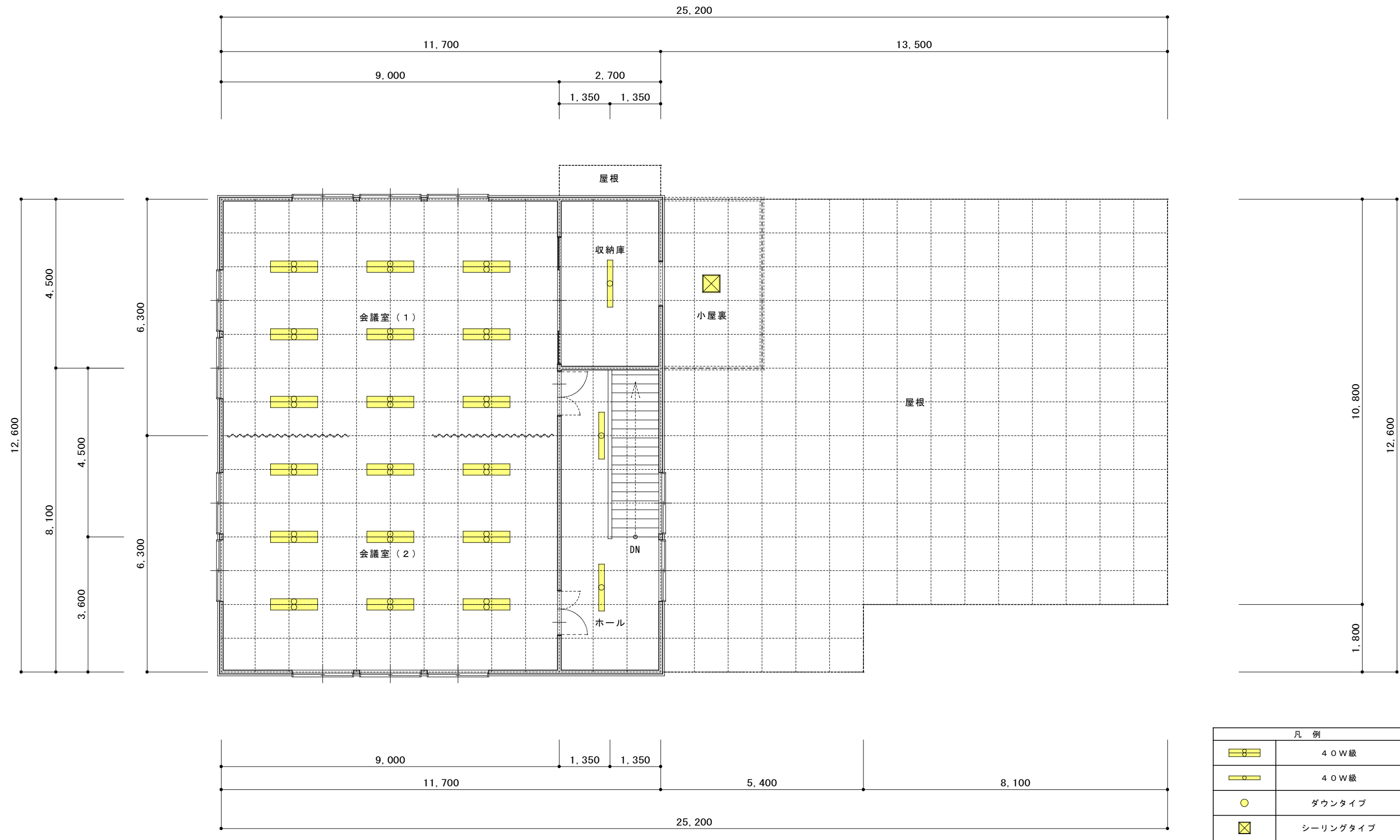
－ 2 階平面図－
